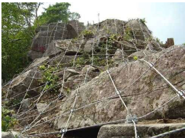
ケーブルネット工(金網なし)
