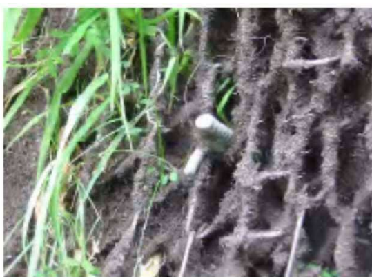
SK厚ネット仕様の植生状況(客土吹付併用)
