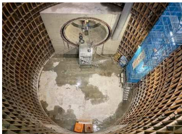
発進立坑内状況
