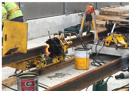
レール敷設状況
