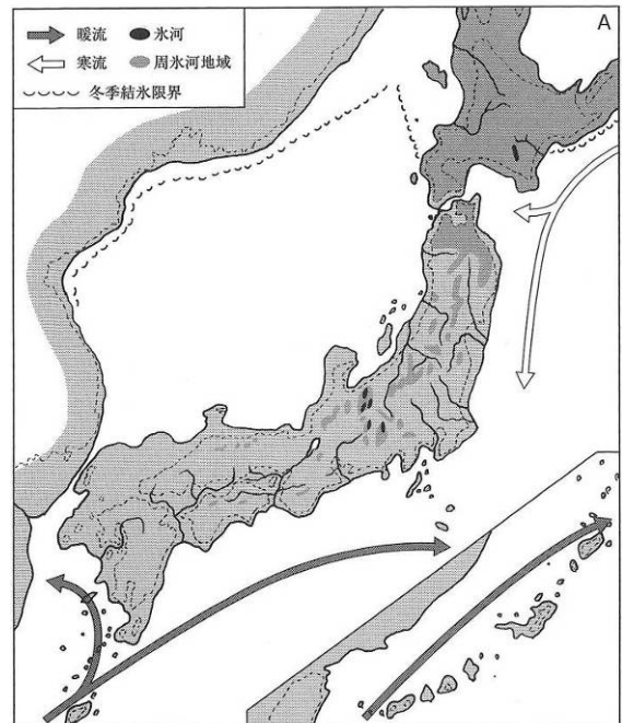
最終氷期（約2万年前）の日本列島付近の海岸線 出典：3)
