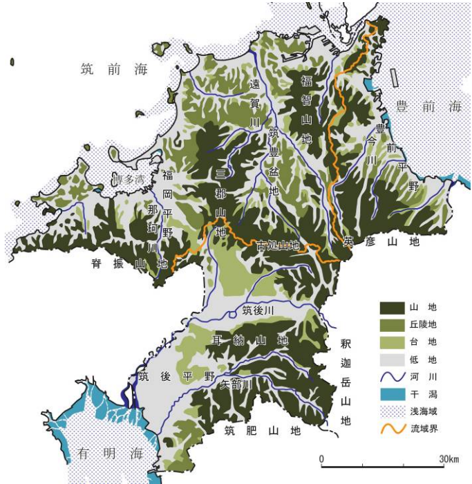
福岡県の地形区分図
