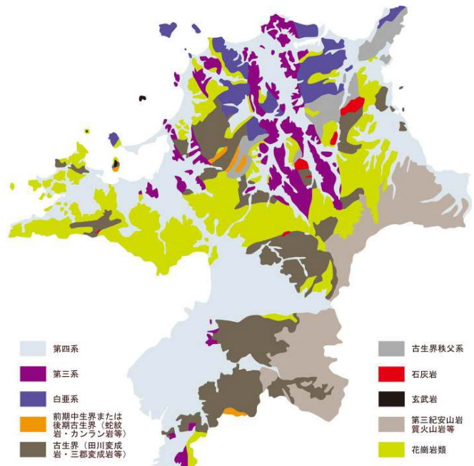
福岡県の地質略図
