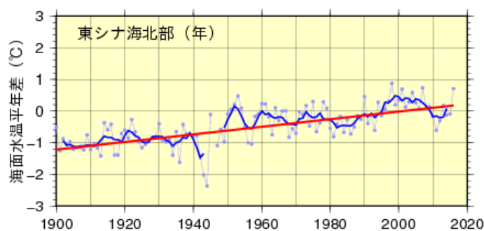
東シナ海北部の海域平均海面水温（年平均）の推移
