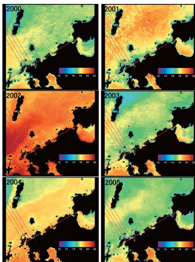
九州北部海域の5月の平均海水温の分布 出典：6)
