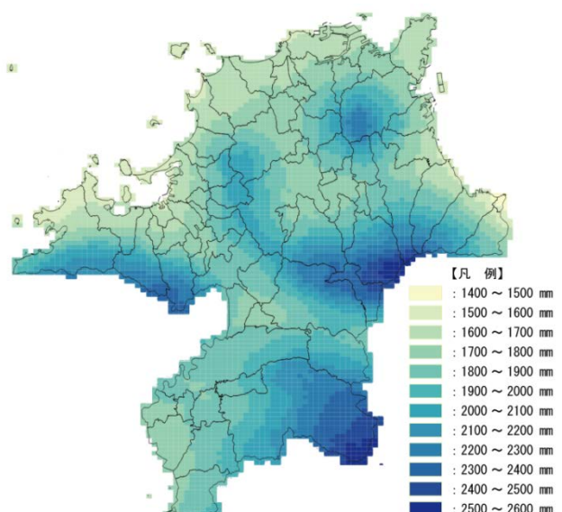
年平均降水量のメッシュ地図
