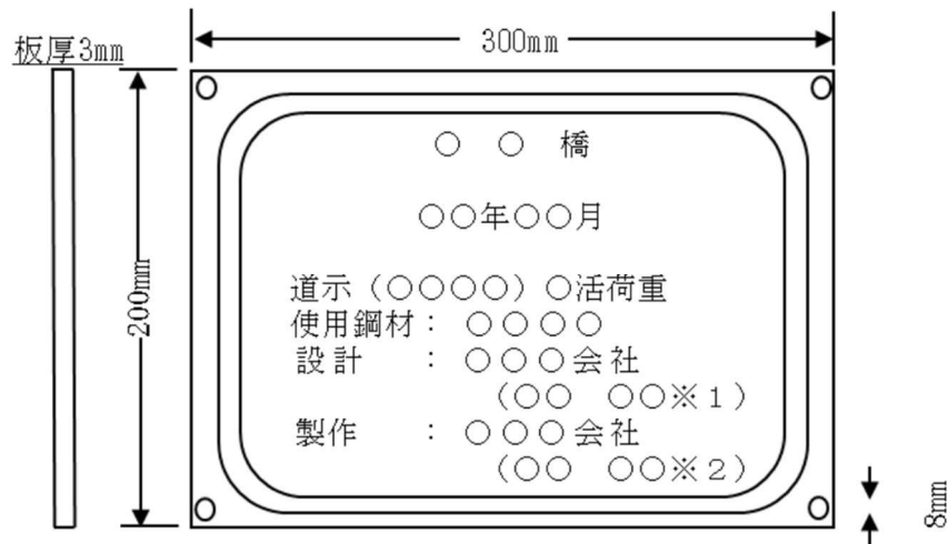
図 10-1-1 銘板の寸法及び記載事項
