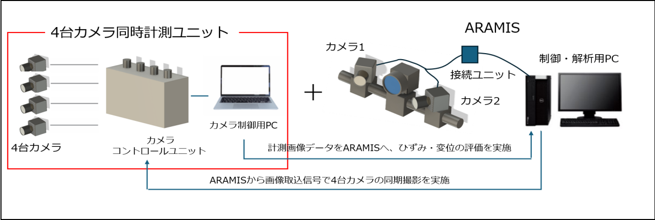
装置構成概略図
