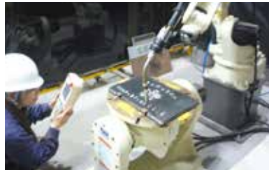
ロボット溶接作業
